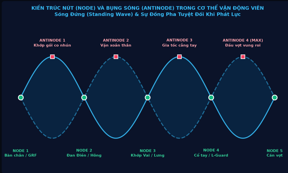
Hình 3: Sơ đồ phân bố các Nút sóng đứng (vị trí ổn định nạp áp suất) và Bụng sóng (biên độ dao động gia tốc cực đại) trong chu trình vung vợt hiện đại.
